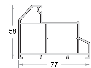
Door Frame Code No : DPDF - 7758
