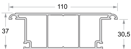
Door Mullion Code No : DPDS - 11037
