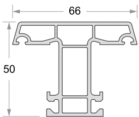
Sash / Mullion Code No : DP - 552
