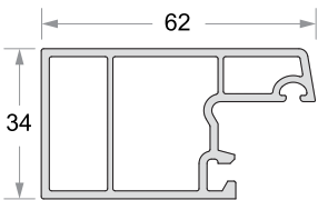
Sash / Style Code No : DP - 601
