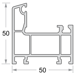
Casement Frame Code No : DP - 551
