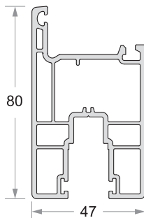
Sliding Door Sash Code No : DP - 704
