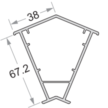
Corner Coupler 135° Code No : DP - 712
