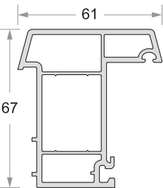
False Mullion Code No : DP - 757
