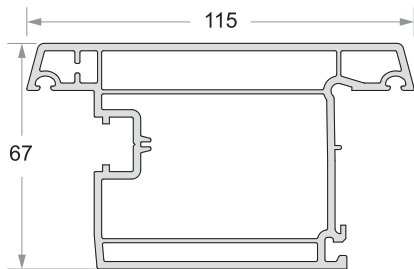
Door Sash Code No : DP - 756
