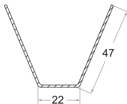
Corner Coupler 135° Code No : ST - 712
