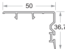
Window Interlock Code No : DP - 705
