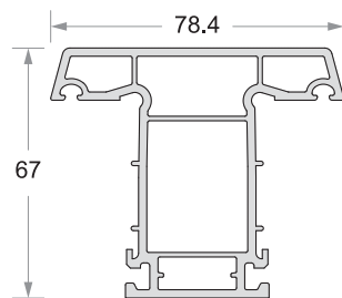
Sash / Mullion Code No : DP - 752
