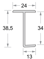
'T' Profile Code No : DP - 602
