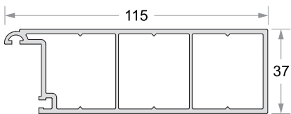
Door Sash Code No : DPDS - 11537
