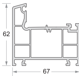
Casement Frame Code No : DP - 751
