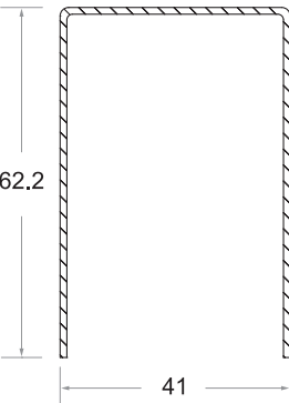
Door Sash Code No : ST - 756
