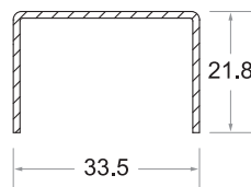
Door Sash Code No : ST - 704
