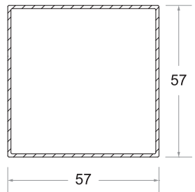
Corner Coupler 90° Code No : ST - 711
