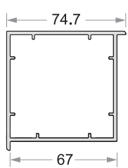
Corner Coupler 90° Code No : DP - 711
