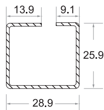
Casement Frame Code No : ST - 751
